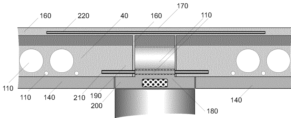
fig 11 cut a-a
