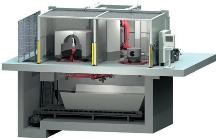
Новейшее поколение линии по производству монолитных колец с днищем – Primuss 2.0
