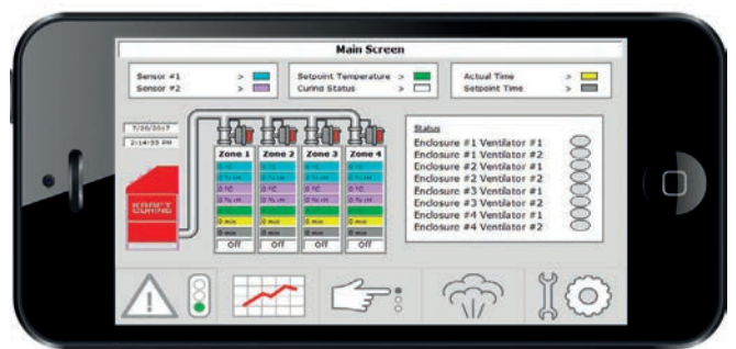
La interfaz Access Anywhere refleja los datos gráficos que normalmente estarían disponibles solo en una pantalla de la empresa
