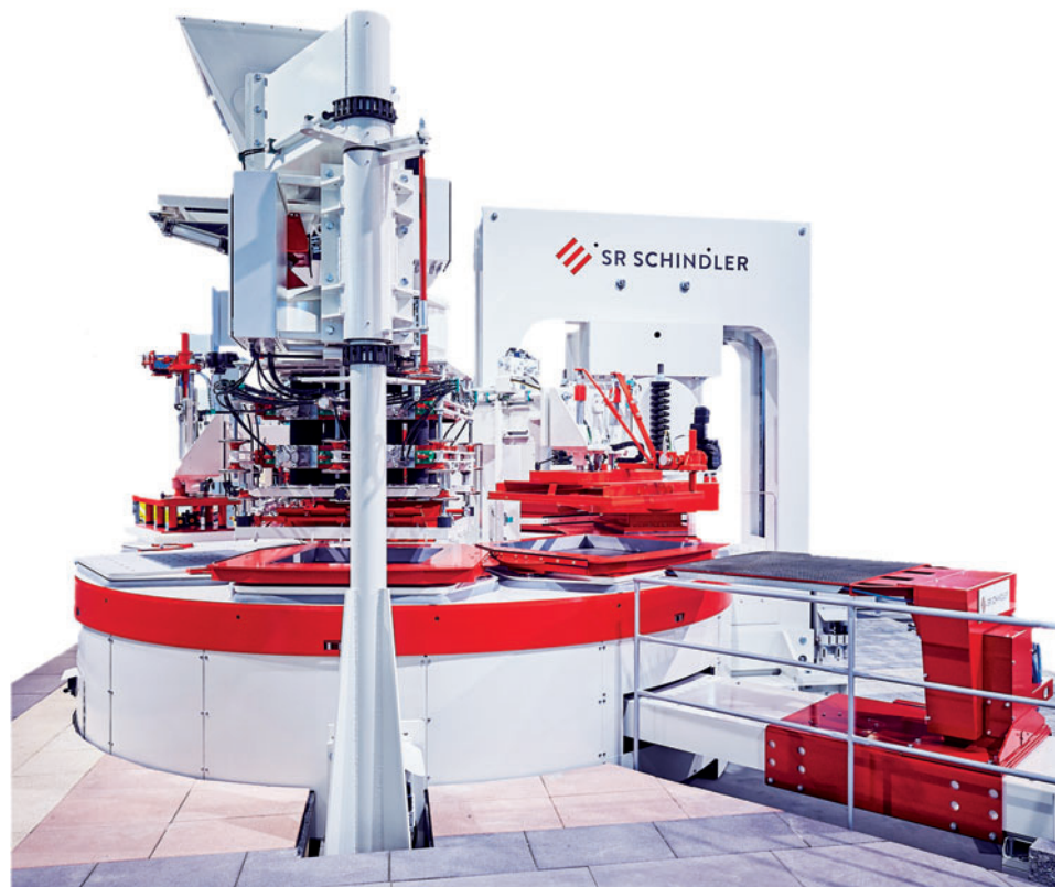
Рис. 4: Герметичный пресс SR Schindler Uni 1200
