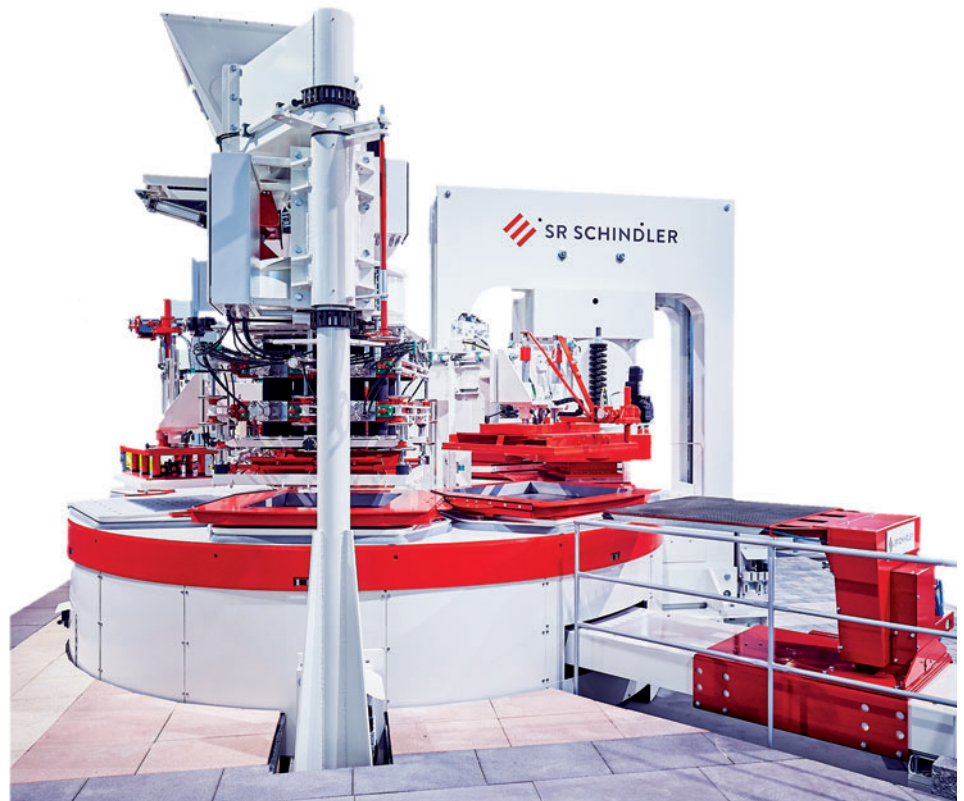
Abb. 4: SR Schindler Hermetikpresse Uni 1200
