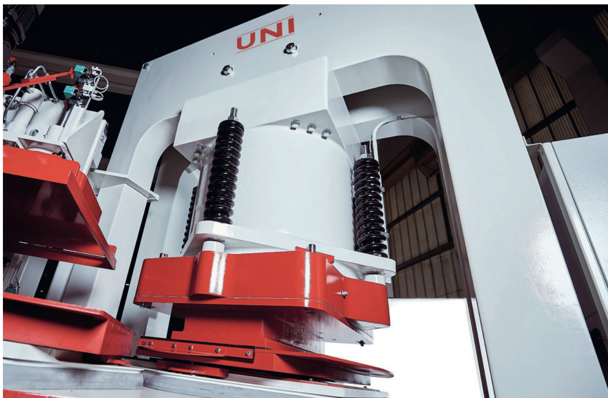
Компания SR-Schindler представила новый пресс типа UNI 1200 в 2019 году на выставке bauma в Мюнхене
