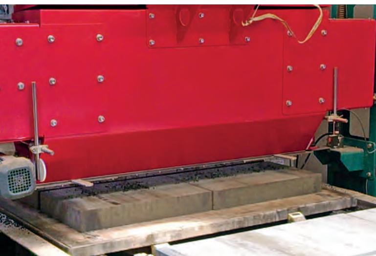
Дозатор T-Rex равномерно распределяет заранее отмеренное количество гранулята по поверхности изделий
