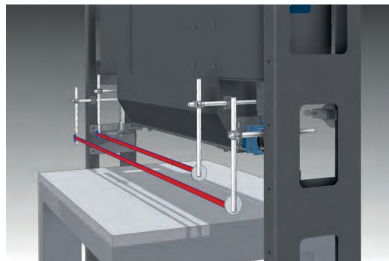
Фоторелейные барьеры распознают приближающиеся изделия и запускают процесс дозирования
