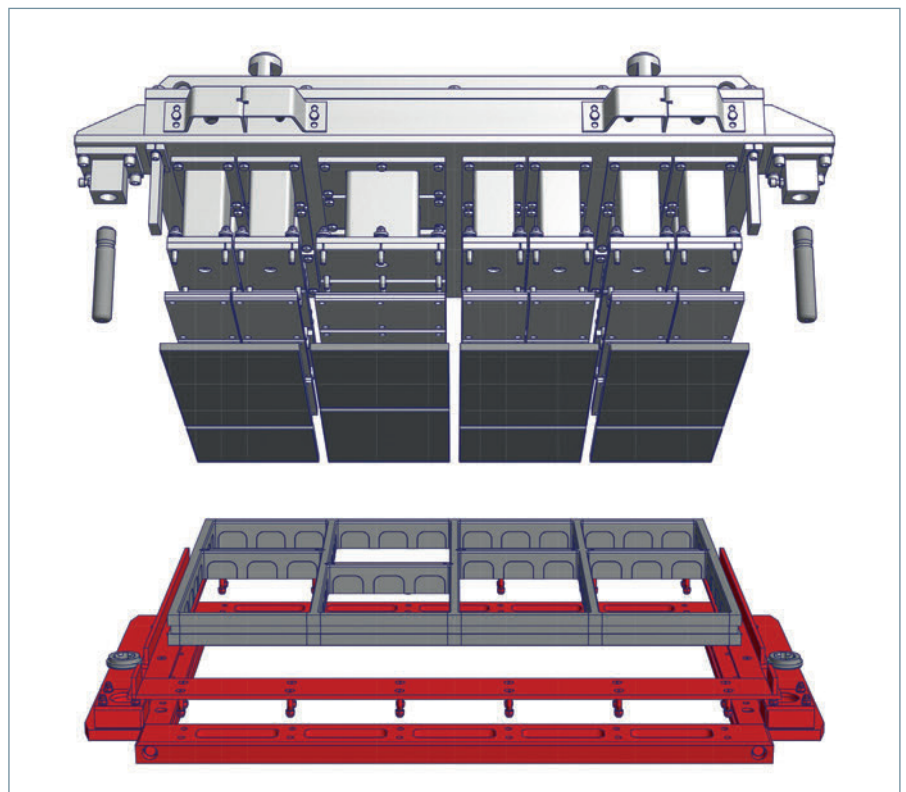
Покомпонентный чертеж формы для бетонных блоков
