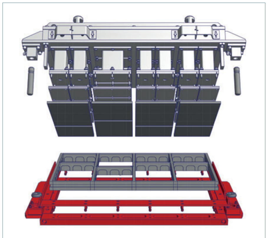
Vista de despiece de un molde para bloques de hormigón
