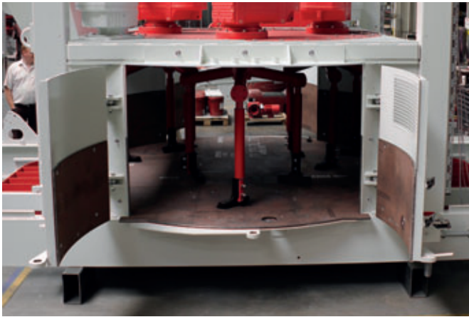
Große Türen ermöglichen die Mischerreinigung von außen.
