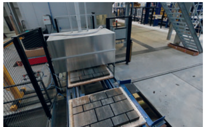
Die frischen Produkte durchlaufen auf der Nasseite eine Sprühanlage für den optionalen Auftrag einer Oberflächenbeschichtung
