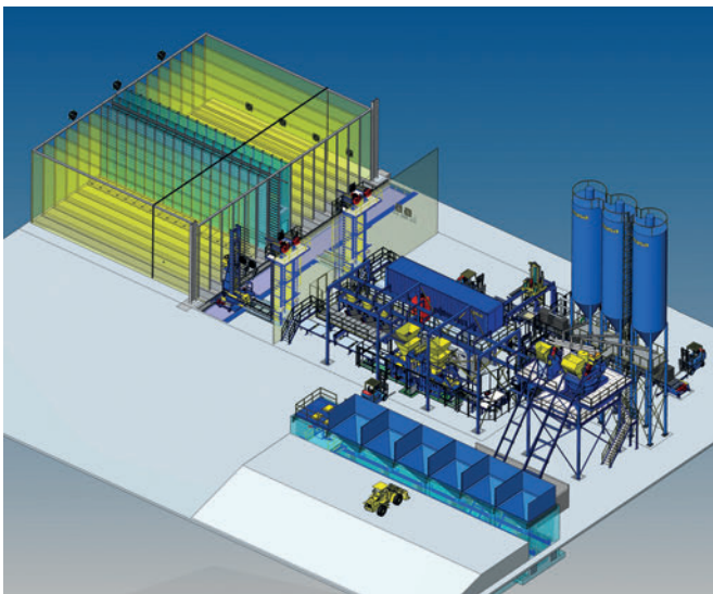
3-D модель завода Masa в Таифе
