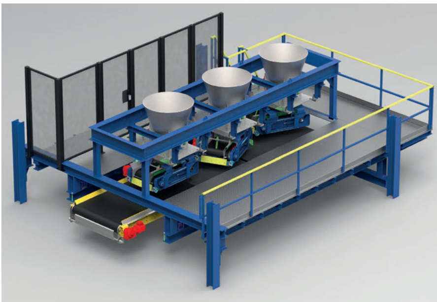
3-D модель новой системы Masa для производства бетонных блоков с цветной поверхностью
