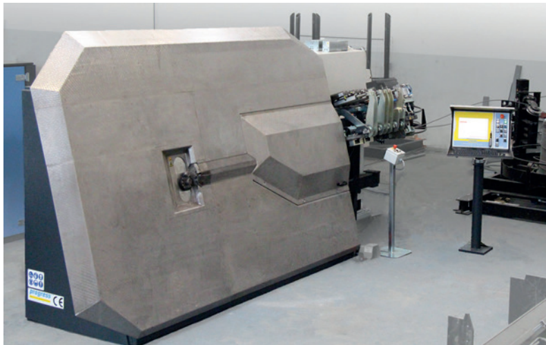
Гибочный автомат фирмы progress Maschinen & Automation
