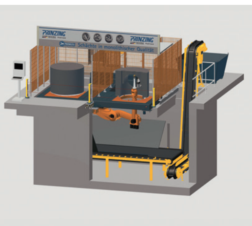
Двойная фрезерная роботизированная станция (монтируется в приямок)
