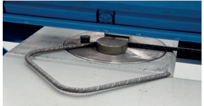
Fig. 2: El Banco de doblado integrado 2BK puede curvar barras de hasta 12 m de longitud.
