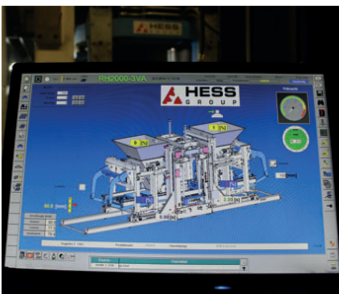
Desde la sala de control se pueden supervisar directamente todos los procesos de producción de las máquinas bloqueadoras RH 2000-3 MVA
