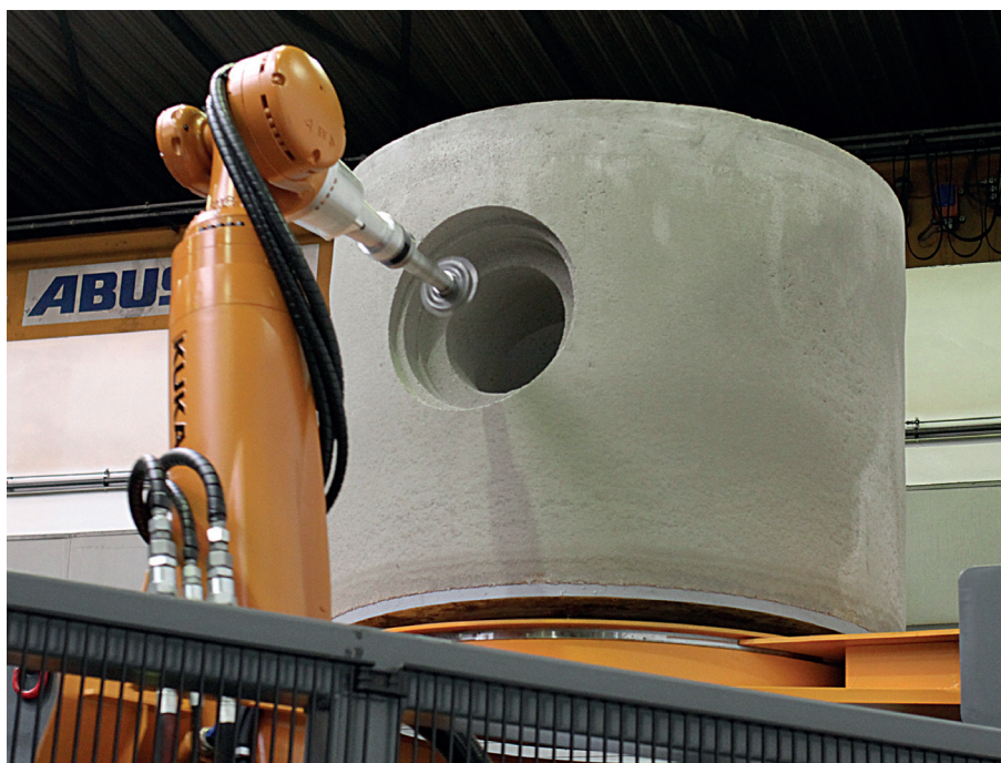
Фрезерный станок по бетону Primuss с точностью до миллиметра фрезерует лотки в монолитных кольцах с днищем
