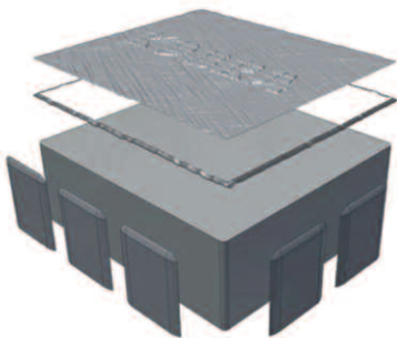
Общая схема производства бетонного камня: формооснастка, фаска и поверхность
