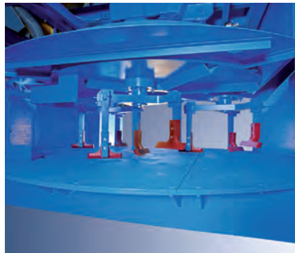
Горизонтальный принудительный бетоносмеситель Masa, тип PH
