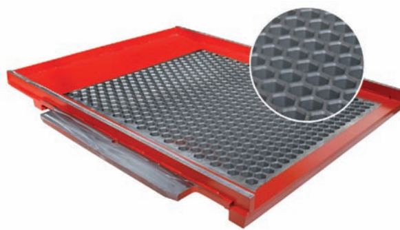
Разнообразие сферы применения форм для бетонных камней – 527-секционная форма для минибрусчатки, основанная на использовании вторичных заполнителей
