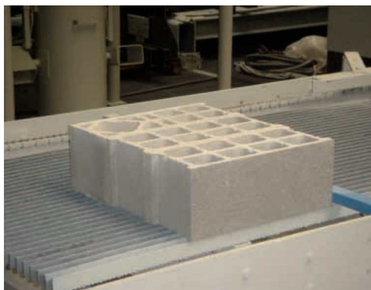
«Гвоздем» выставочной программы стала презентация новой установки Cutmaster, которая будет более подробно представлена на страницах следующего выпуска журнала «Международное бетонное производство». Cutmaster позволяет изготавливать стеновые камни с идеально ровной поверхностью для укладки при помощи энергосберегающей технологии с заменой толстого слоя раствора на тонкий слой мастики.
