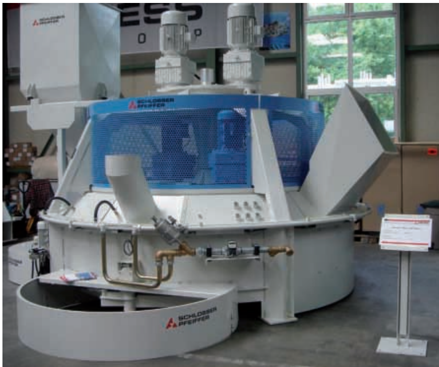
Смеситель типа Тур SM 3000-2 был представлен на домашней выставке в новом модульном исполнении, что позволяет поставлять его в более короткие сроки и по более выгодной цене
